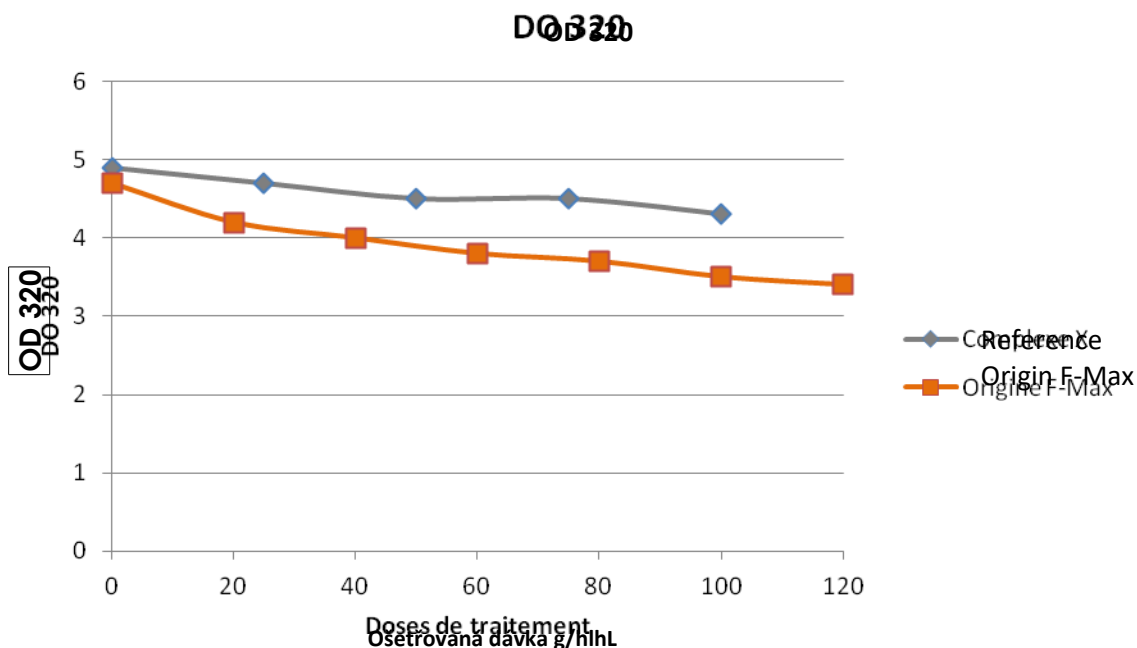
Graf 1: Účinek přípravku ORIGIN F-MAX na koncentraci oxidovatelných sloučenin (OD 320)
